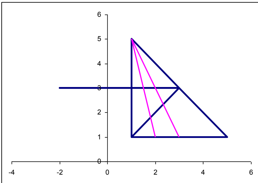
Рис.6 Изображён прямоугольный равнобедренный тр-к. Длина катета равна 4 ед. Из прямого угла опущена высота на гипотенузу. Высота затем переходит в среднюю линию тр-ка. Из верхней вершины тр-ка проведены две сиреневые линии, делящие основание на отрезочки длиной 1, 1 и 2 ед. Смысл сиреневых линий такой же, как и жёлтых линий на рис. 3. Верхнюю вершину тр-ка обозначим К, левую – О, правую – Т, середину гипотенузы – L, основания сиреневых линий – R и S. Основание тр-ка изображает плоскость, которую фотографирует самолёт (рис. 3), вершина К – местоположение самолёта, а средняя линия и высота изображают положение
