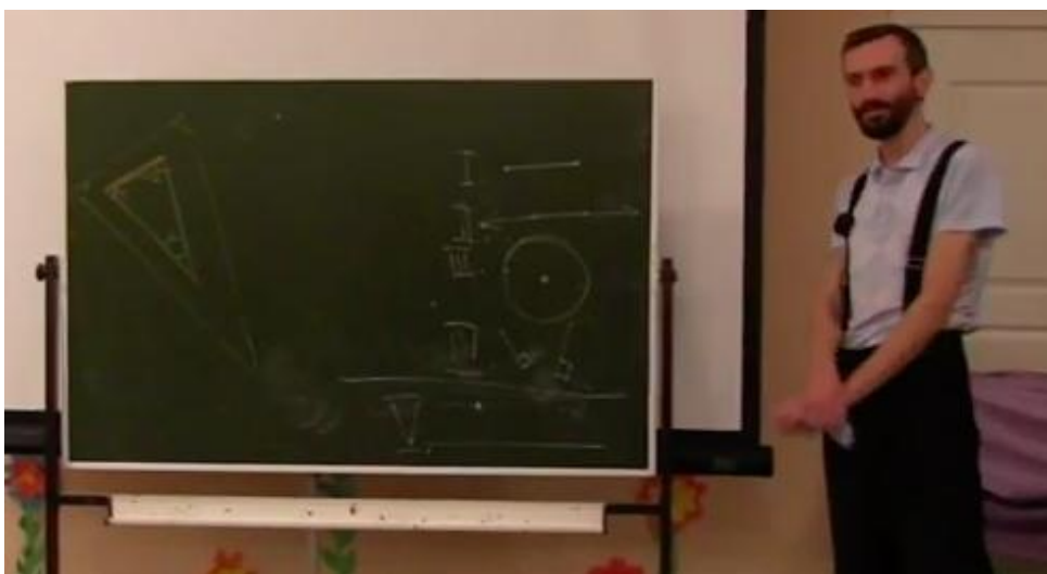
Рис.28 (слева) Тут уж и астрономы призадумались – а у всех ли «космических» треугольников сумма углов равна в точности 180 градусов?
