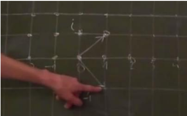
Рис.17 Вот чудеса-то: сумма чисел (1+i) и (1-i) равна их произведению!
