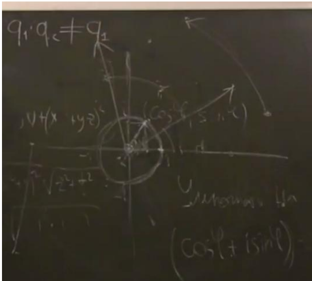
Рис.12 Раскинулось поле по модулю пять, Вдали вектора замелькали... (студенческая песня)
