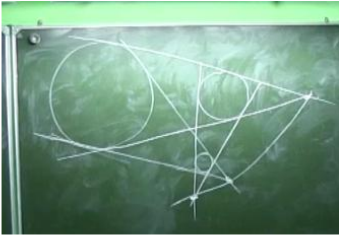
Рис.18 Рисунок-шутка. (Из-за нарочито небрежно нарисованных пар касательных читателю пытаются внушить НЕВЕРНЫЙ вывод о том, лежат ли точки пересечения пар касательных на одной прямой).
