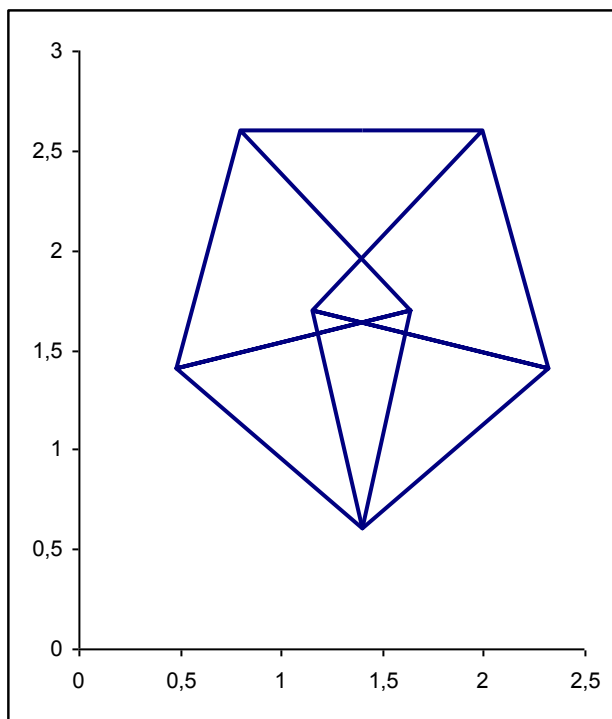
Рис.21 Длина всех рёбер равна 1. Конструкция содержит 7 вершин (точки кажущегося пересечения на оси симметрии (верхние) вершинами не являются).
