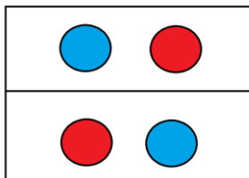
Рис.12 Эти пары для нас не разные, а одинаковые
