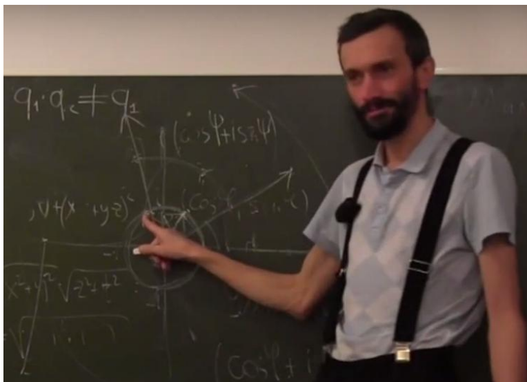
Рис.13 Наступление на комплексные числа закончилось успешно.
