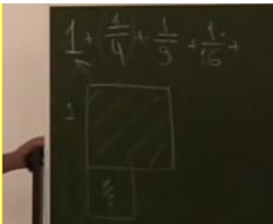
Рис.24 Геометрический смысл исходной суммы.
