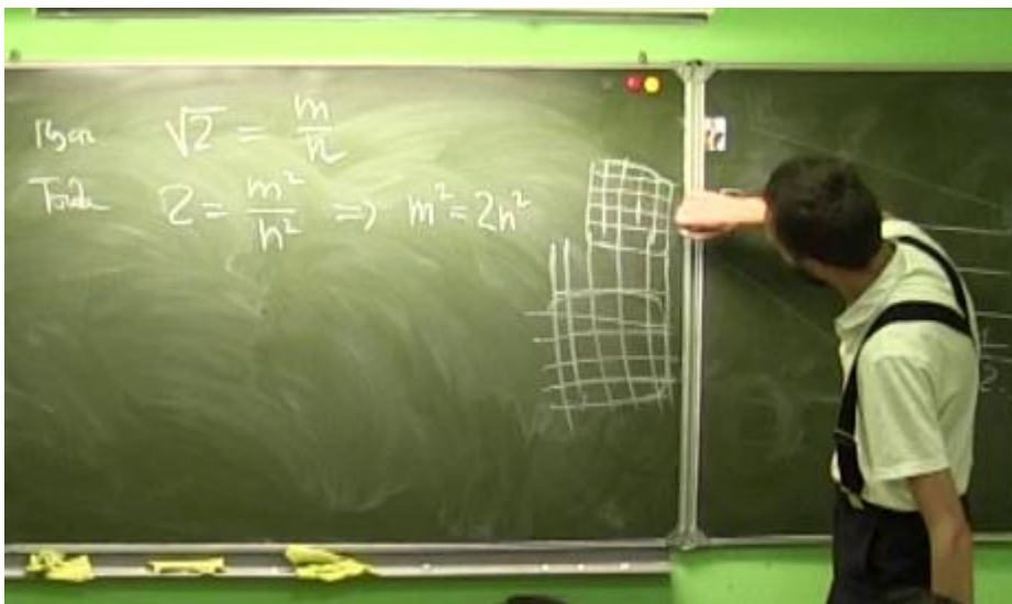
Рис.15 Что-то не получается нарисовать два таких квадрата. И это — неспроста!
