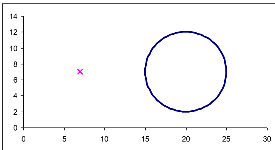
Рис.14 Веди прямые «туда, не знаю куда» и построй касательную.
