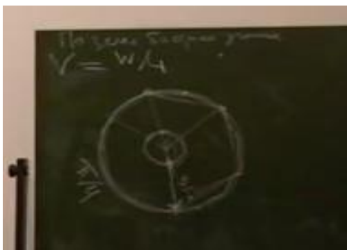
Рис.23 Почему \pi больше трёх.
