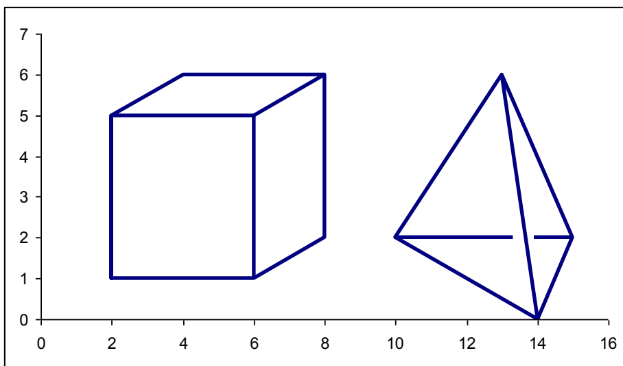
Рис.26 Слева – куб (невидимые линии не изображены), справа – тетраэдр из проволоки.
