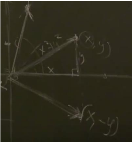
Рис.7 Внимание: над вектором написано «корень( x^2 + y^2 )», а не x^2 + y^2 .
