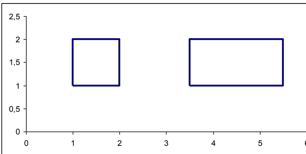
Рис.1 Два разных фазовых пространства.
