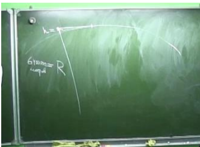
Рис.3 Земля в разрезе. Расстояние от центра до вершины горы R+h , расстояние от центра до точки касания R . Через L обозначено расстояние от вершины до точки касания.
