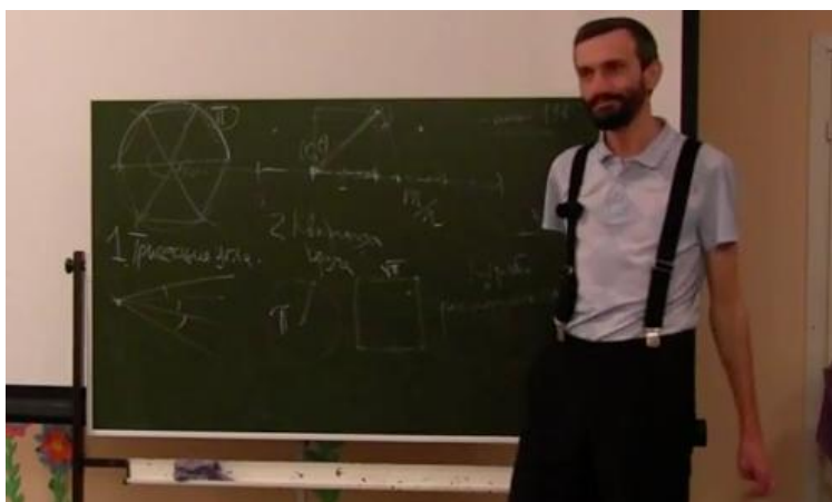
Рис.8 Слева сверху: как строить 6-угольник. Слева внизу: задача о трисекции угла. Посередине сверху: соединяя линейкой противоположные вершины единичного квадрата, строим НЕ РАЦИОНАЛЬНОЕ число «корень из двух».
