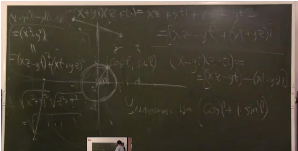
Рис.11 И на Земле, и в ближнем космосе справедливы эти формулы...
