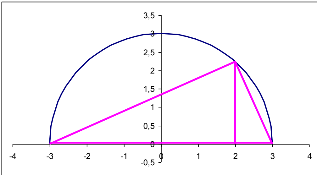
Рис.10 Отрезок a=5 отложен между x=-3 и x=2 ; единичный отрезок – между x=2 и x=3 . Строим полуокружность радиуса 3. Проводим перпендикуляр из точки x=2 . Это и есть отрезок длины \sqrt{5} . Все три сиреневых треугольника прямоугольные, и все они подобны друг другу.
