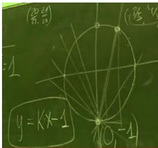
Рис.5 Обратите внимание на вспомогательный прямоугольный треугольник справа с вершиной в точке (0, -1) .
