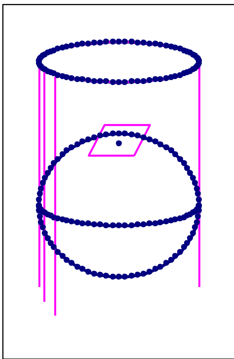
Рис.10 Поверхность Земли с указанием экватора и Северного полюса (нижняя часть рисунка). Красные вертикальные линии – образующие бесконечной в обе стороны цилиндрической поверхности. Для удобства восприятия верхняя часть цилиндрической поверхности срезана горизонтальной плоскостью (верхняя синяя линия – край среза). Отдельная синяя точка – это Северный полюс. Через него проведена горизонтальная плоскость, касающаяся Земли. Эта плоскость схематически изображена в виде красного параллелограмма.
