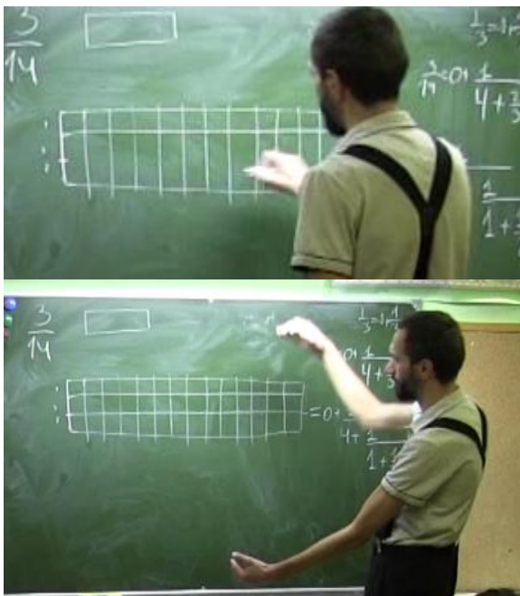
Рис.4 Вот такие будут кусочки, если разделить поровну 3 яблока на 14 ребят!
