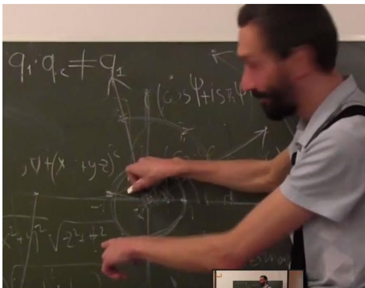
Рис.14 Комплексные числа – это большое чудо. Но и мелкие чудеса комплексных чисел заслуживают нашего внимания. Например, прямо с неба падают формулы «синус суммы» и «косинус суммы».
