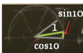
Рис.12 \sin 10^\circ построить нельзя. Это вам не какой-нибудь \sin 72^\circ !
