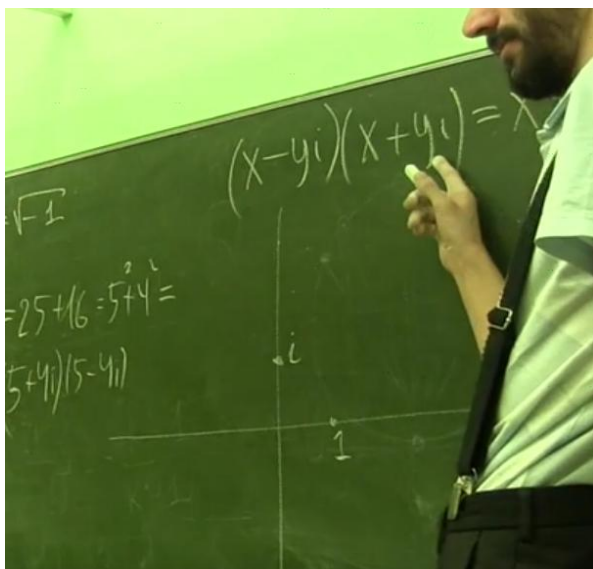
Рис. 7 Вот где притаилось загадочное число i .
